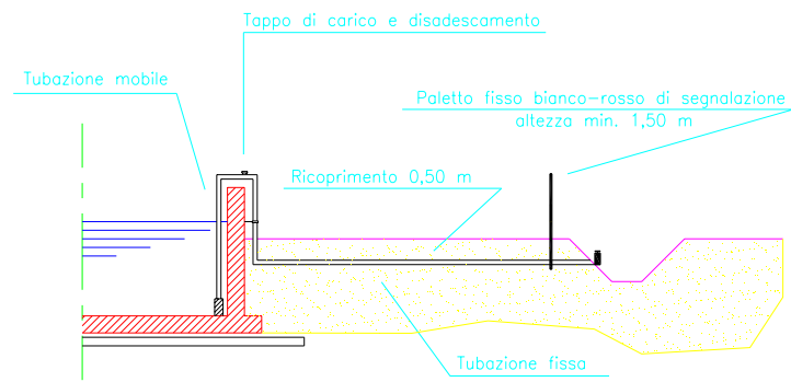
B2. Canale a sezione rettangolare – sponda in destra idraulica
